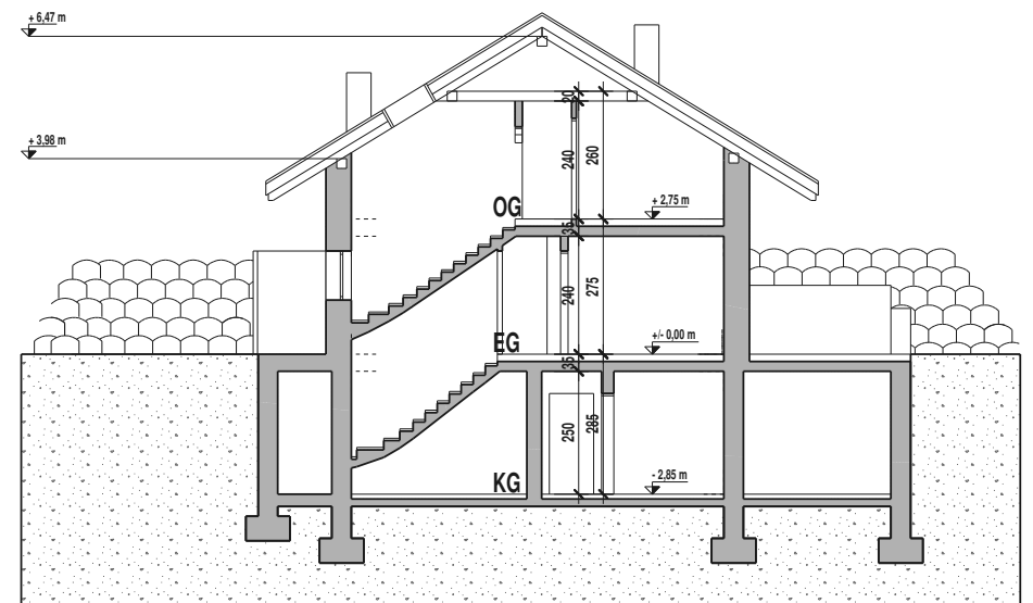
Sezione - Section
