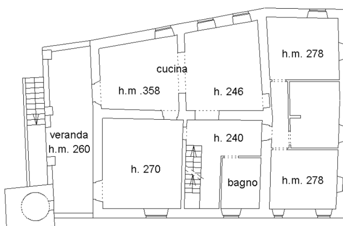
PIANO PRIMO
